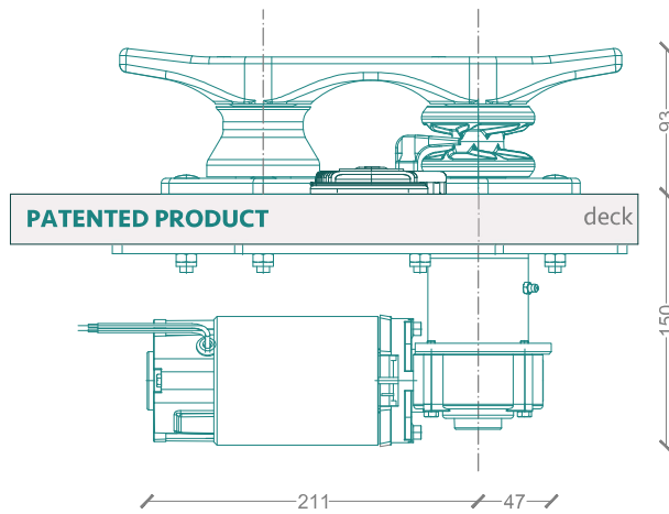
LONGITUDINAL SECTION
